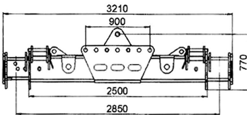
Traverse in Transportstellung
