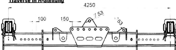
Traverse in H-Stellung
