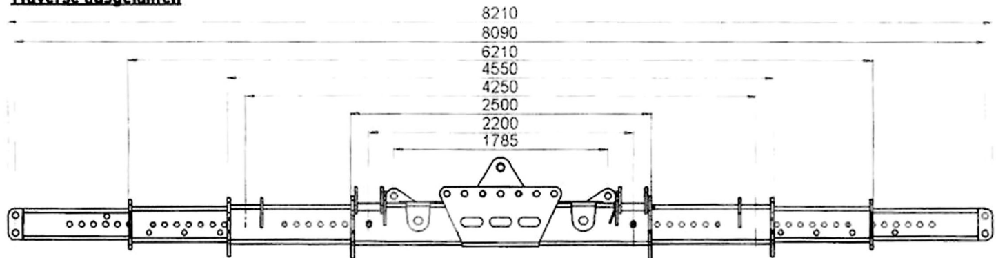
Traverse ausgefahren
